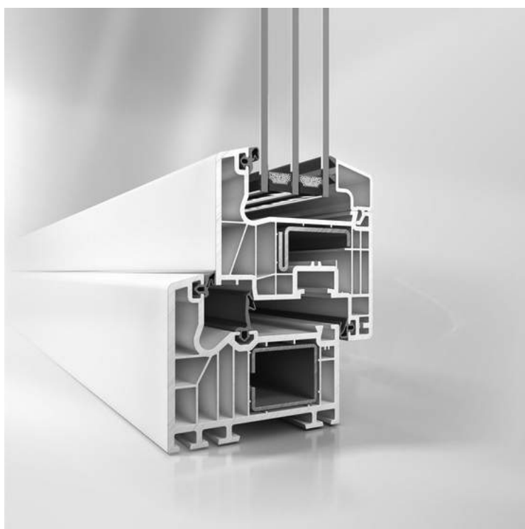
SCHÜCO Portes et fenêtres PVC CORONA SI 82
